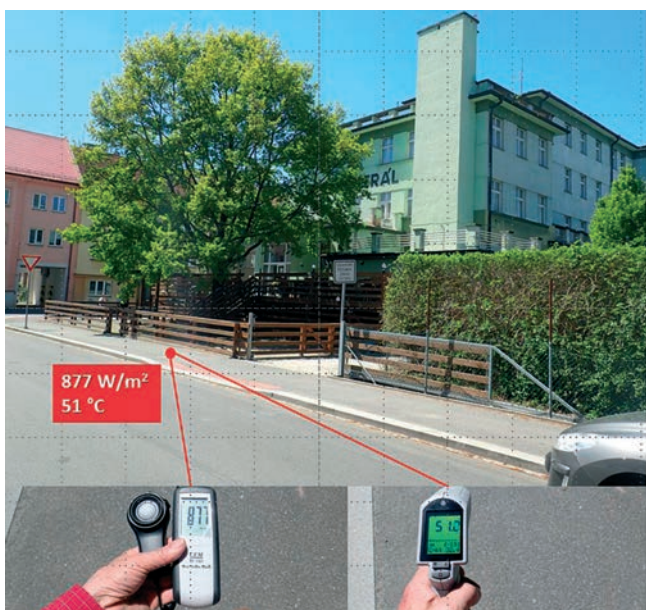
Obř. 1: Na 1 m 2 chodníku dopadá 877 W sluneční energie a povrchová teplota je 51 °C. Ve stínu stromu je povrchová teplota 26,9 °C a na 1 m 2 dopadá 82 W sluneční energie. Strom vypaří 20 litrů vody za hodinu a chladí výkonem cca 14 kW, fotosyntézou strom do biomasy váže přibližně 0,02 kW
