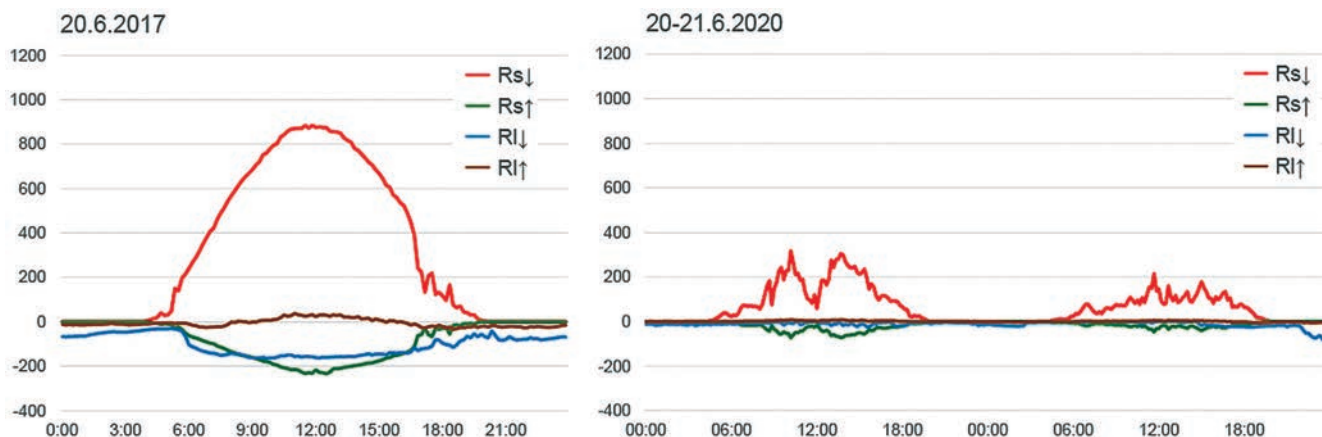
Obr. 14: Denní chod přicházejícího ( RS \downarrow ) a odraženého ( RS \uparrow ) slunečního záření ( W \cdot m^{-2} ) a dlouhovlnného/tepelného záření mezi čidlem a oblohou ( RI \downarrow ) a dále mezi čidlem a povrchem země ( RI \uparrow ) v letním slunovratu při jasné obloze 19.–20. 6. 2017 (vlevo) a v letním slunovratu při zatažené obloze 20.–21. 6. 2020 (vpravo) [Jirka, et al., 2021]
